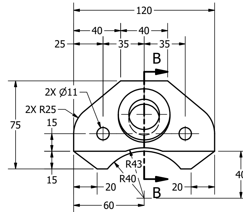
GUIDE SCALE 1 / 2
