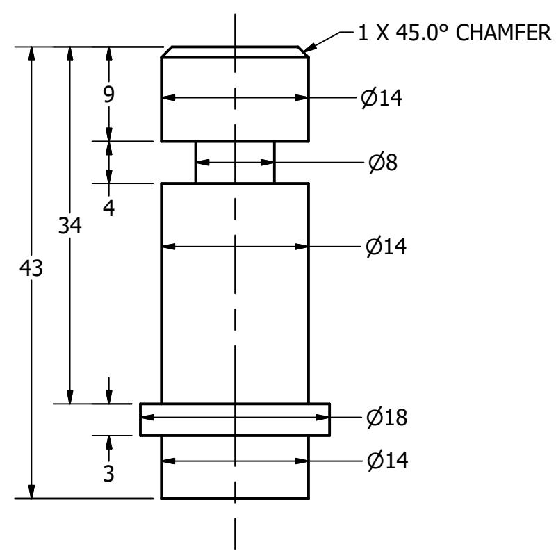
POST SCALE 2 : 1
