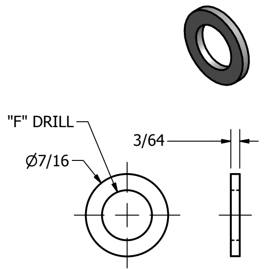
WASHER SCALE 2 : 1
