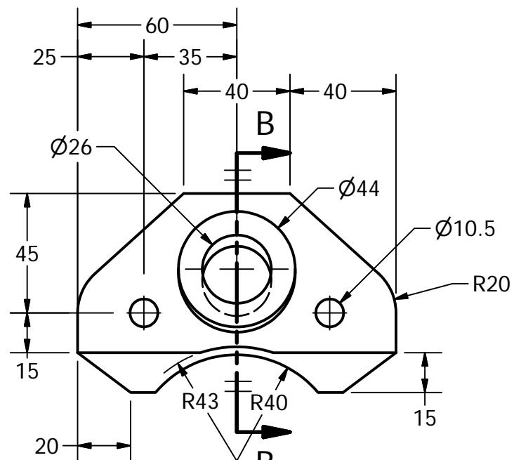
GUIDE SCALE 1:2
