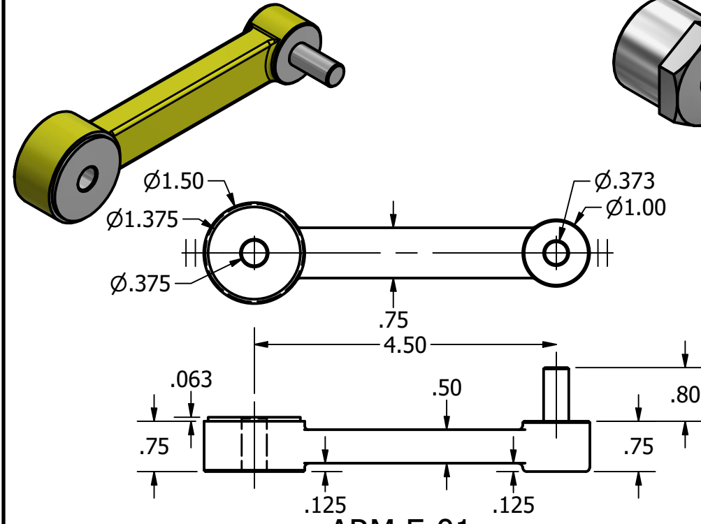
ARM E-01 SCALE 1:2
