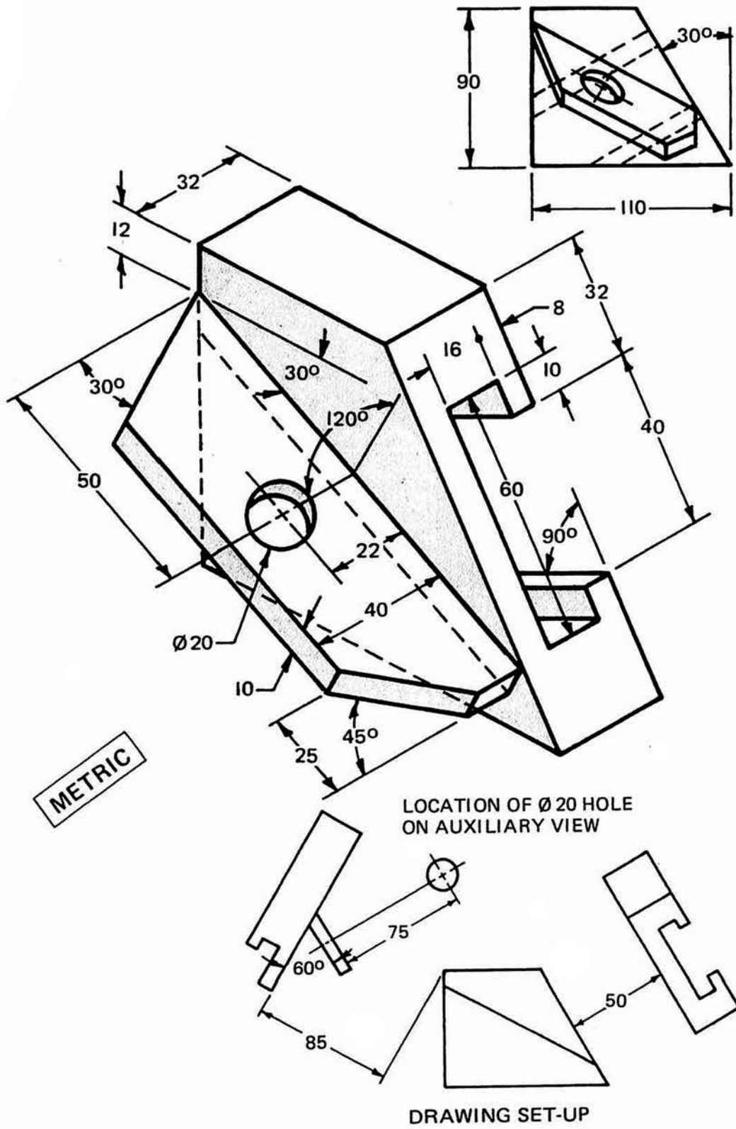
Fig. 7-60 Pivot arm.
