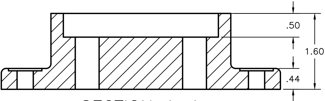
SECTION A-A
