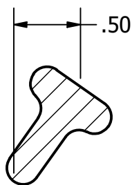
SECTION D-D SCALE 1 : 1
